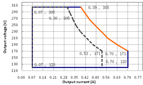
LUP-120X305Z
