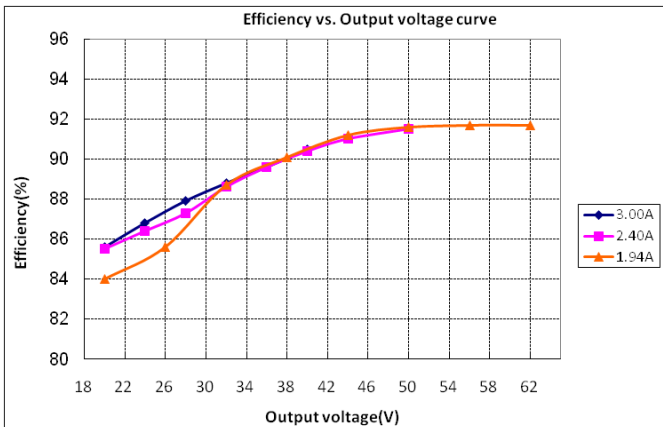
LUP-120X170Z (Vin=115Vac)
