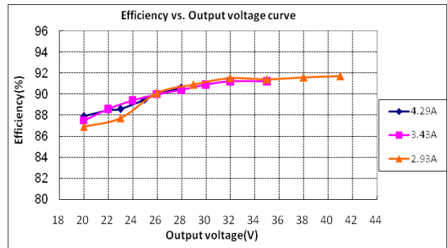
LUP-120X041Z (Vin=230Vac)
