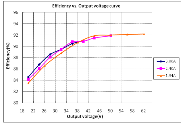
LUP-120X170Z (Vin=230Vac)
