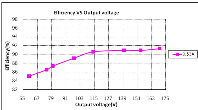
LUP-120X170Z (Vin=115Vac)
