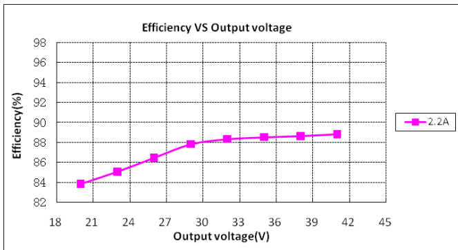
LUP-120X041Z (Vin=115Vac)
