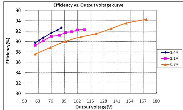
LUP-120X170Z (Vin=230Vac)
