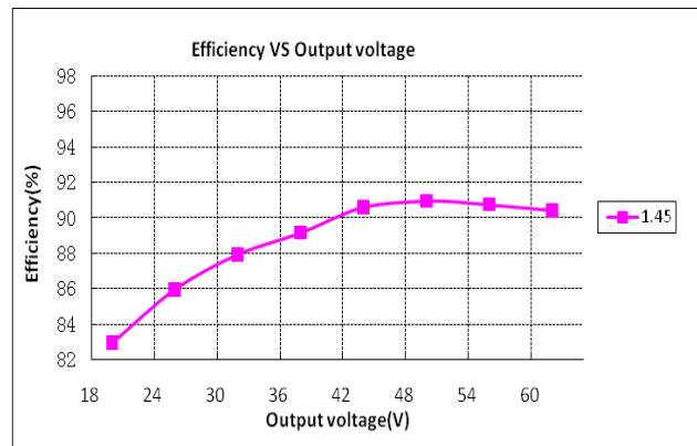
LUP-120X062Z (Vin=277Vac)
