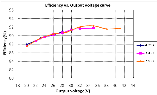
LUP-120X062Z (Vin=230Vac)
