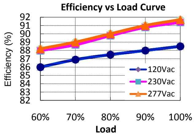
MTP-240X054( I_o=5.72A )
