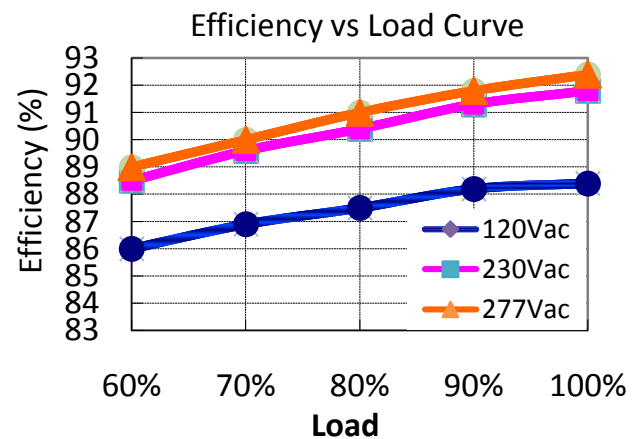
MTP-240X068( I_o=4.2A )
