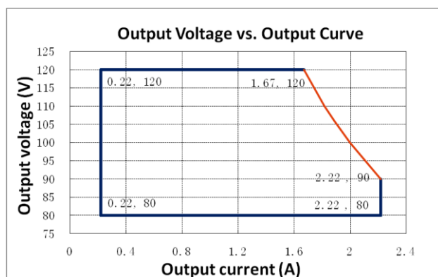
LDP-200X305 -B
