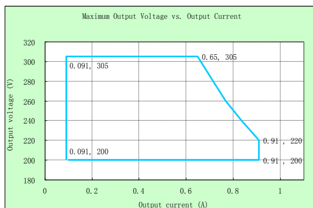
LDP-200X305 -B
