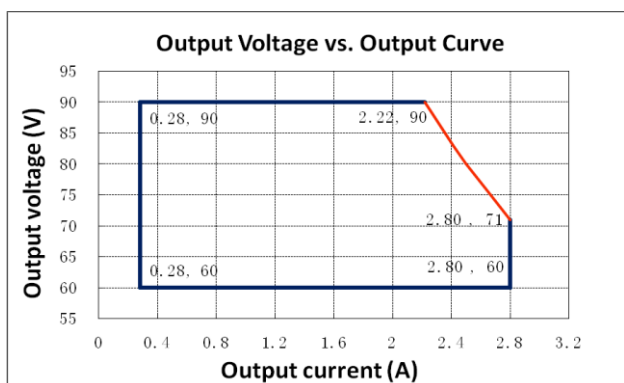
LDP-200X305 -A
