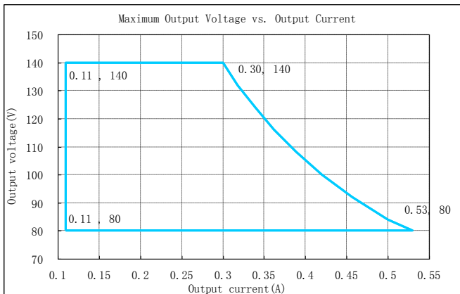
LDP-042X140
