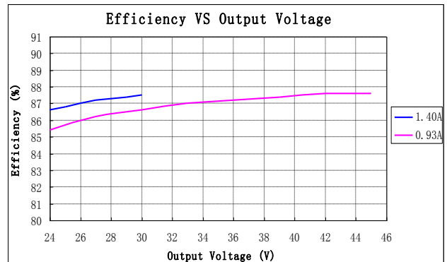
LDP-042X080(Vin=230Vac)
