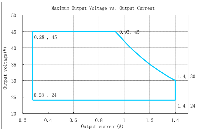
LDP-042X045
