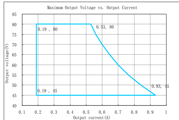
LDP-042X080
