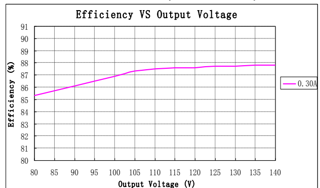
LDP-042X140(Vin=230Vac)
