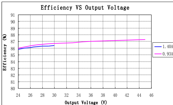
LDP-042X080(Vin=115Vac)
