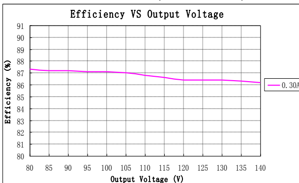
LDP-042X140(Vin=115Vac)
